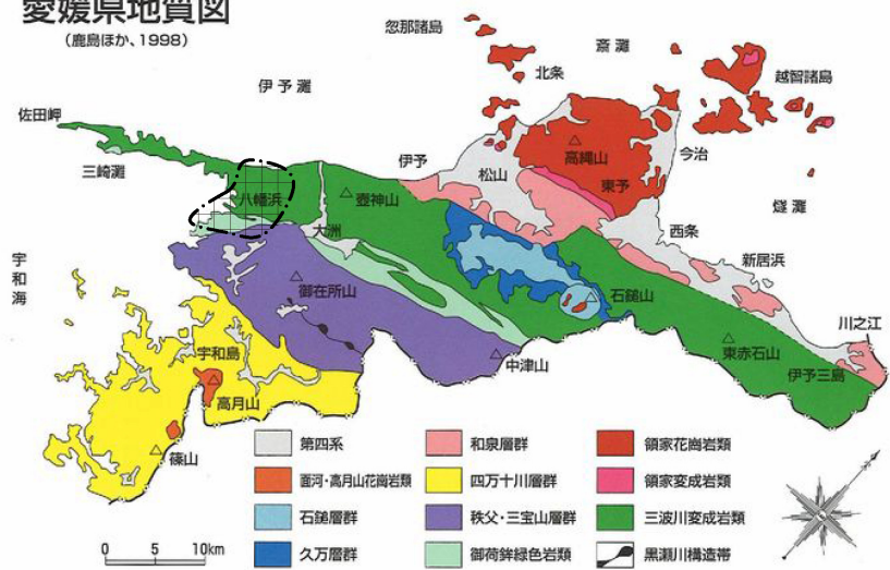
愛媛県地質図
