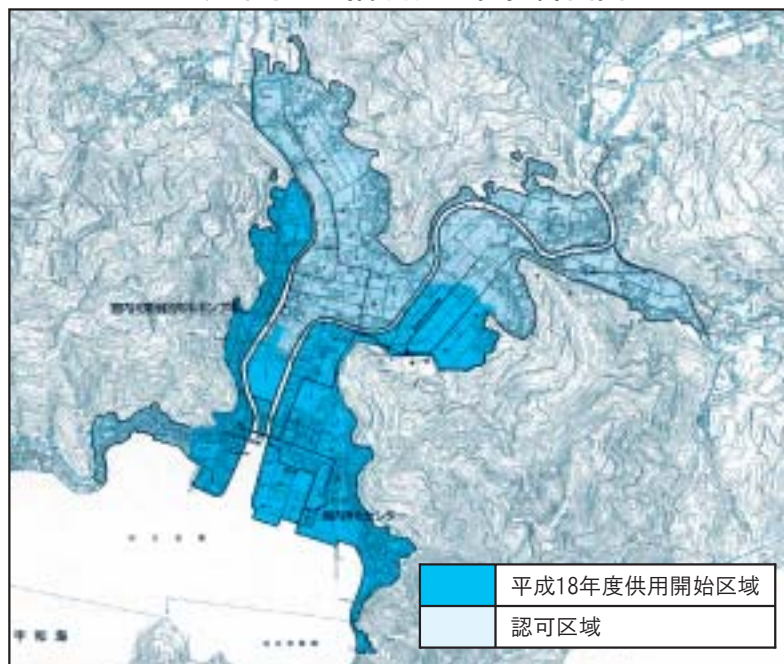
公共下水道（保内処理区）計画図
