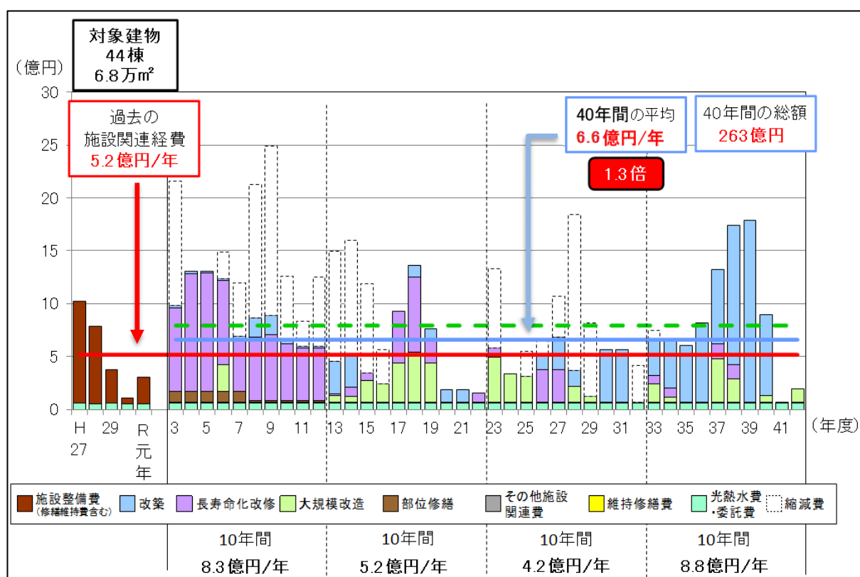
図表 20 更新費用推計グラフ（長寿命化型）
